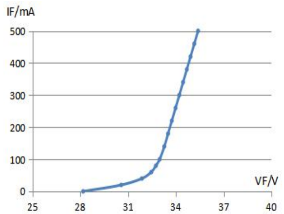
4、伏安特性曲线 Voltage Vs Current
