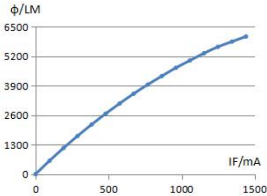
3、电流与光通量曲线图 Current Vs Lumen
