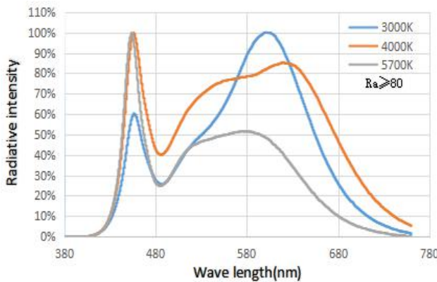
5、相对光谱曲线图 Relative spectral curve
