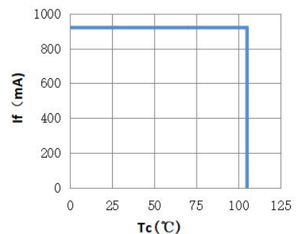
2、Tc-I f 曲线图 TC VS I f curve
